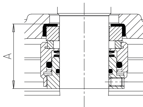
Fig. 17: Medida de montagem A
