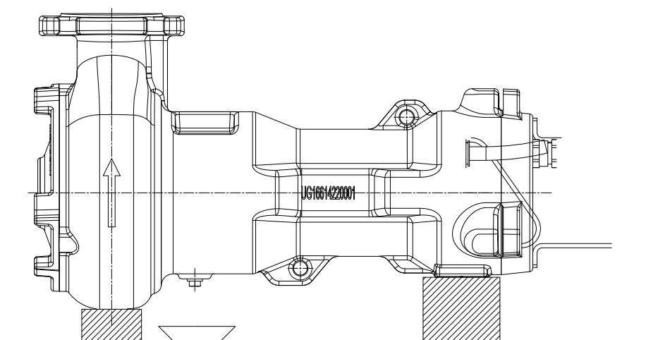
Afb. 14: Smeermiddel aftappen
