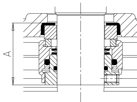
Afb. 17: Inbouwmaat A
