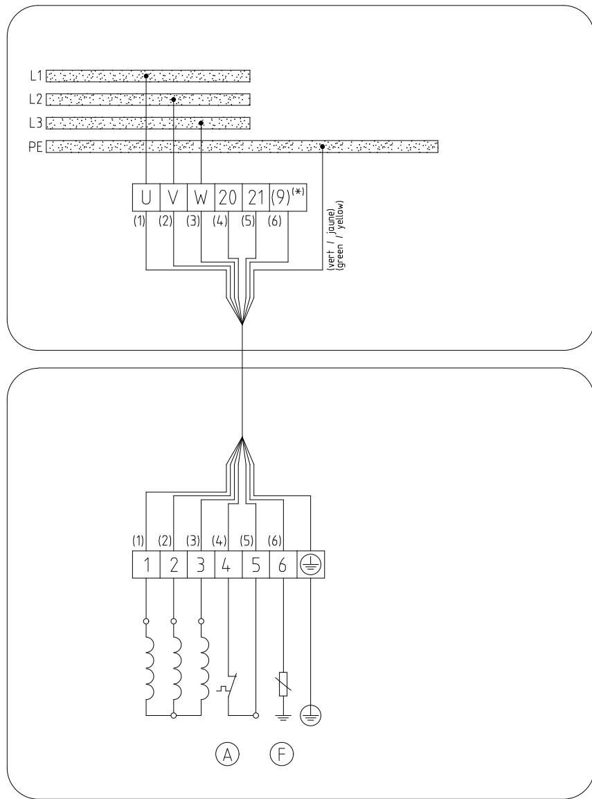
Fig. 22: Plano de conexiones eléctricas, 7G1,5
