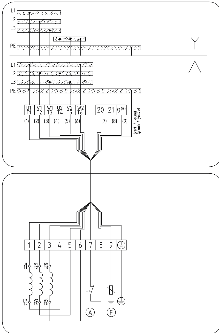
Afb. 24: Elektrisch aansluitschema, 7G1,5 + 3x1 of 7G2,5 + 3x1
