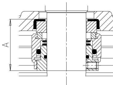
Fig. 17: Medida de montaje A
