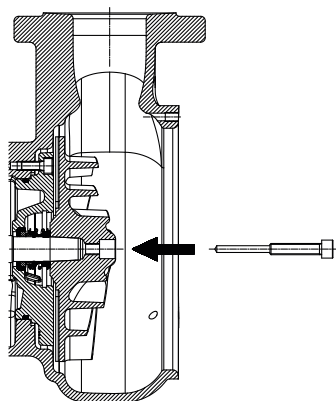
Fig. 16: Parafuso de descompressão
