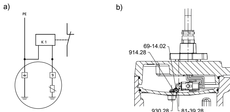
Fig. 11: Ligar o relé para eléctrodos: a) esquema de ligações, b) posição dos eléctrodos no corpo do motor
