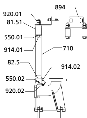
Afb. 8: 2 geleidebuizen monteren
