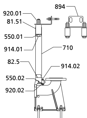
Fig. 8: Montaje de 2 tubos guía
