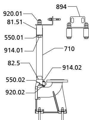
Fig. 8: Montar 2 tubos de guia
