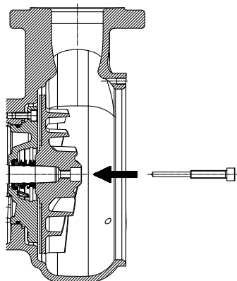
Afb. 16: Afdrukbout
