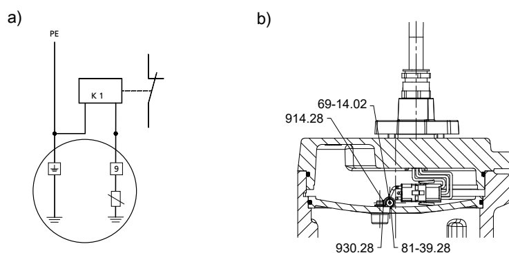
Fig. 11: Conexión del relé de electrodos: a) Esquema de conexiones; b) Posición del electrodo en la carcasa del motor
