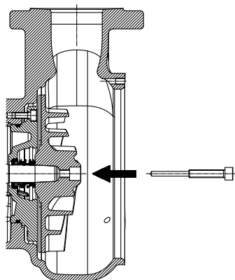
Fig. 16: Tornillo de desmontaje
