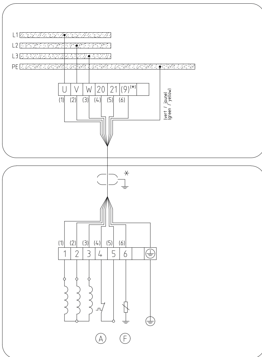
Fig. 23: Esquema de ligações eléctricas: 8G1,5
