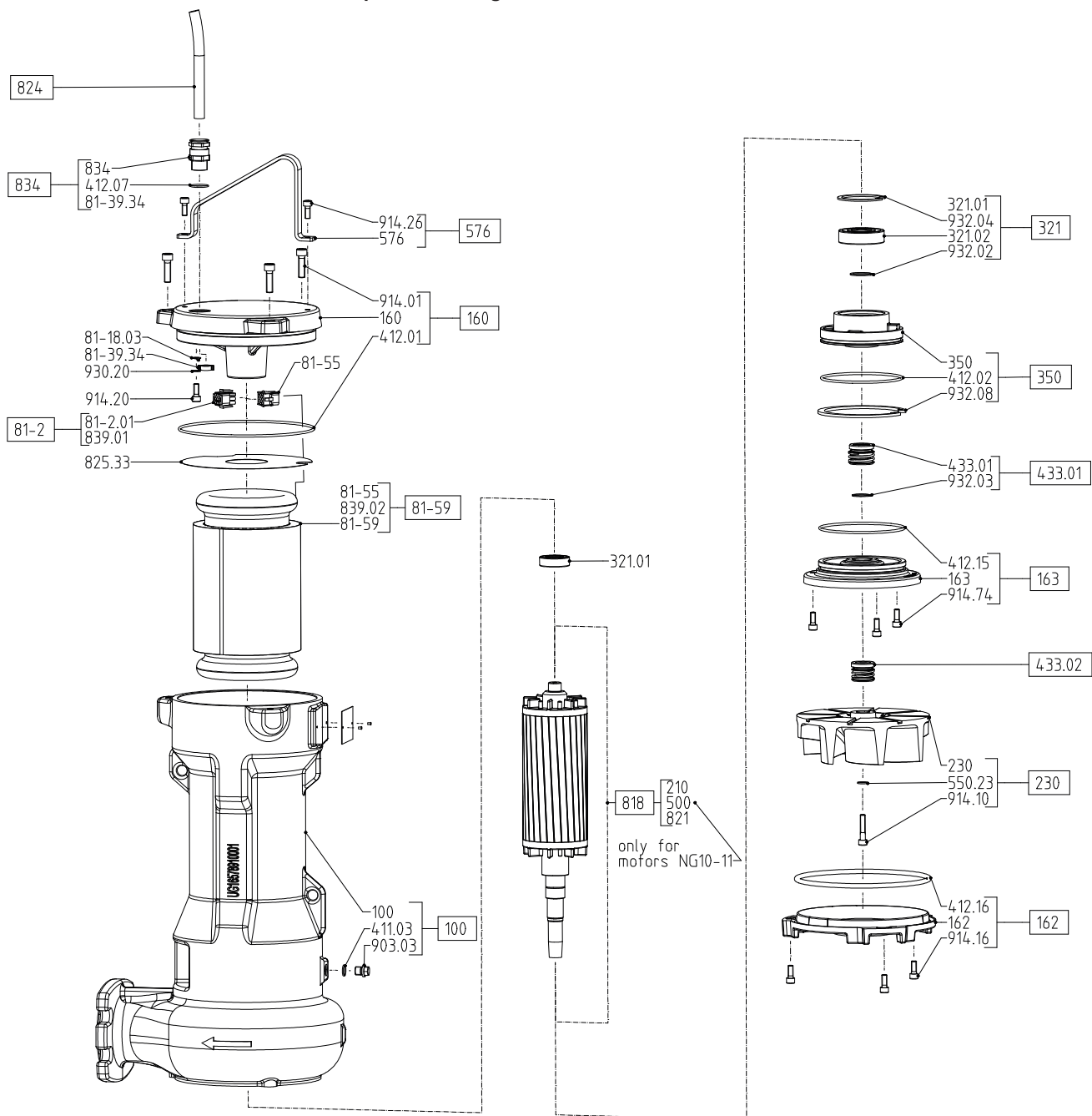
Afb. 20: Explosietekening
