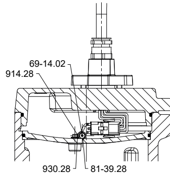
Afb. 11: Elektrodenrelais aansluiten: a) aansluitschema, b) positie van de elektrode in het motorhuis
