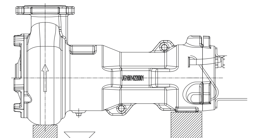
Fig. 14: Purga del líquido lubricante
