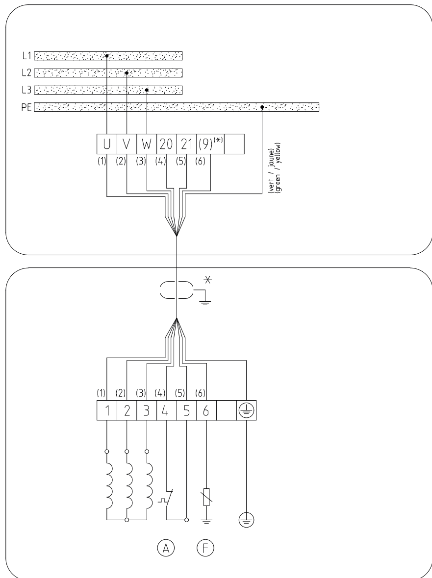
Afb. 23: Elektrisch aansluitschema, 8G1,5
