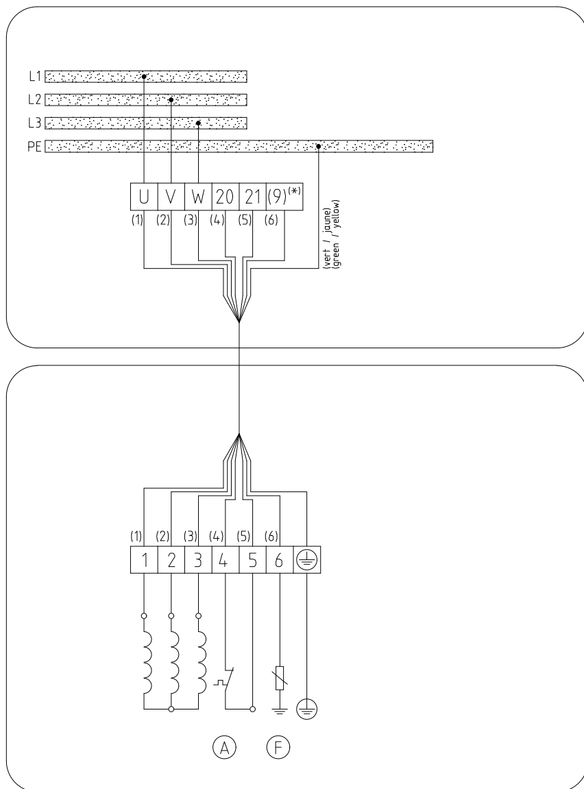
Afb. 22: Elektrisch aansluitschema, 7G1,5
