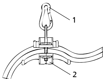
Fig. 12: Fijación de los cables de conexión
