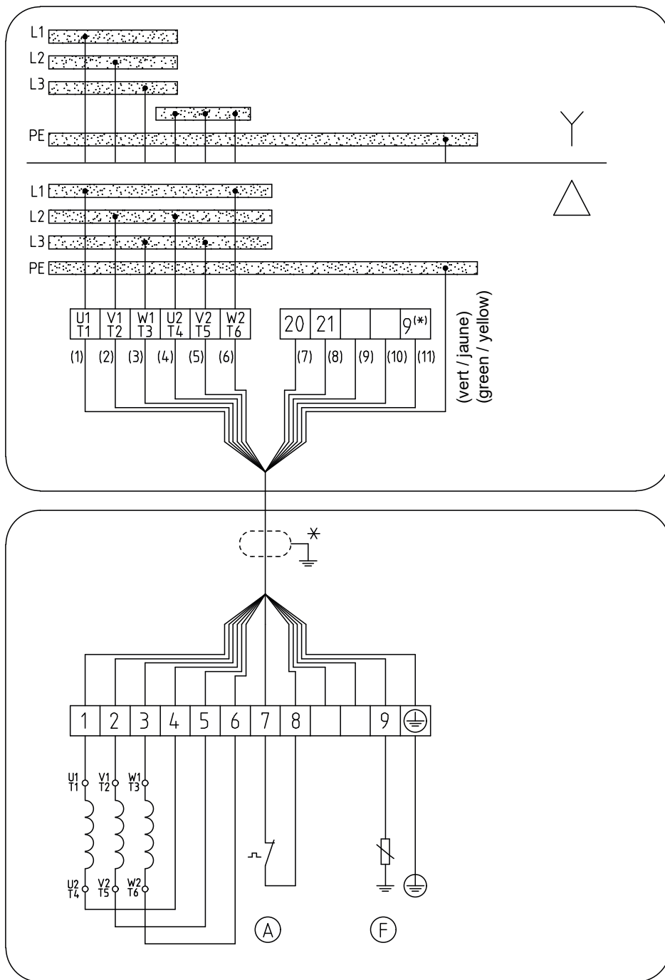
Afb. 25: Elektrisch aansluitschema, 12G1,5 of 12G2,5
