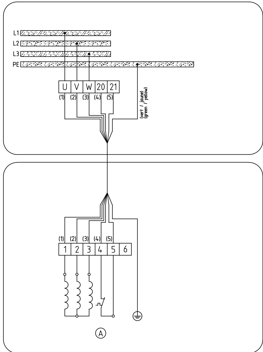
Fig. 21: Plano de conexiones eléctricas, 4G1,5 + 2x1
