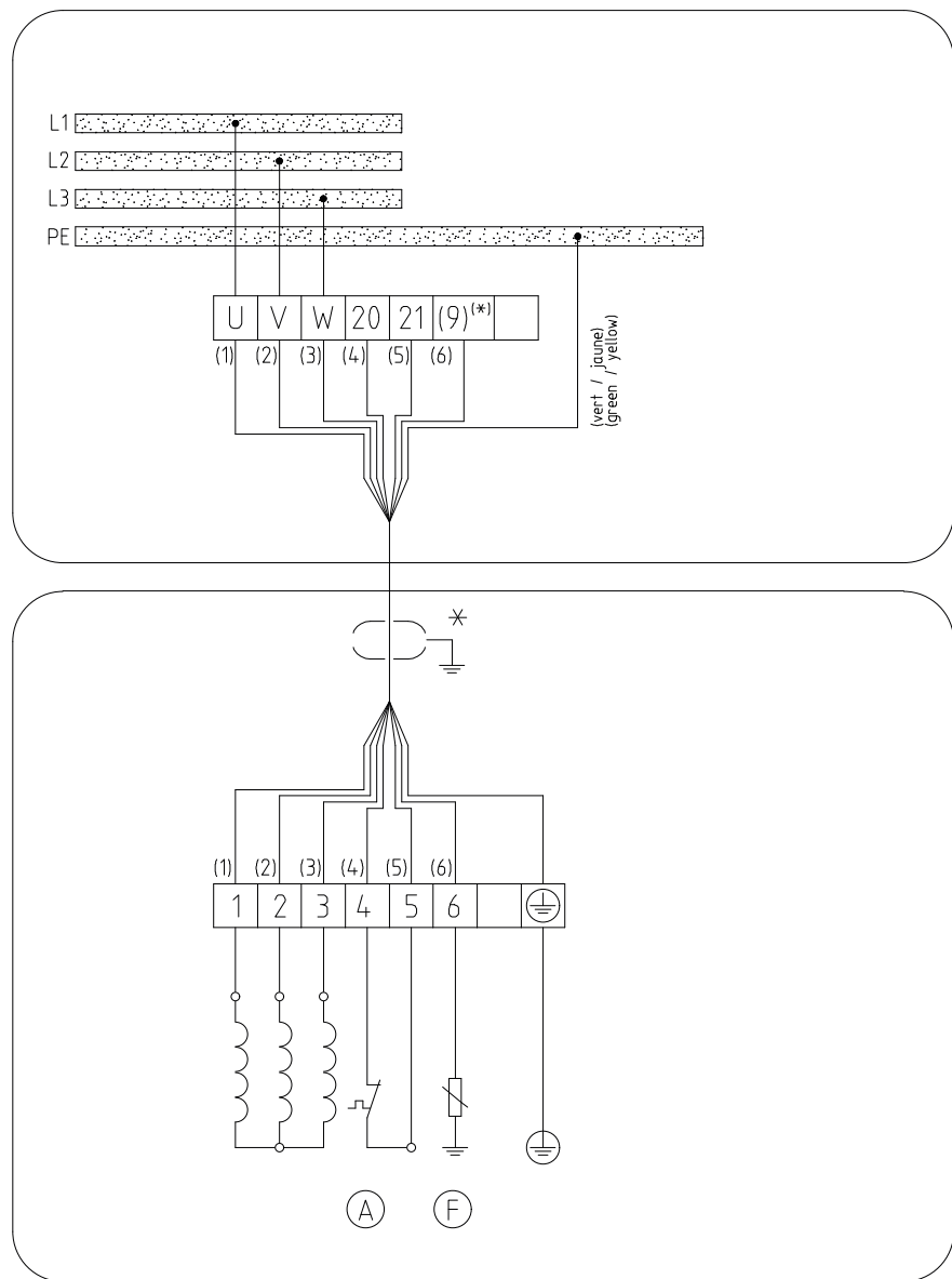
Fig. 23: Plano de conexiones eléctricas, 8G1,5
