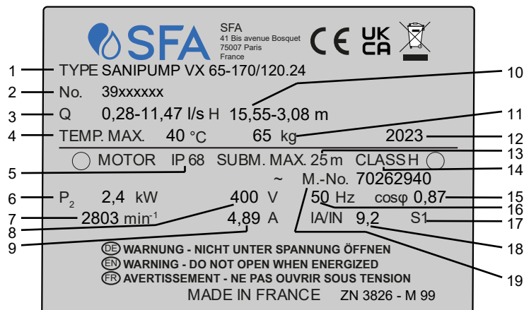
Afb. 1: Typeplaatje (voorbeeld) Standaard-pomppaggregaat
