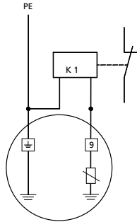
Afb. 11: Elektrodenrelais aansluiten: a) aansluitschema, b) positie van de elektrode in het motorhuis
